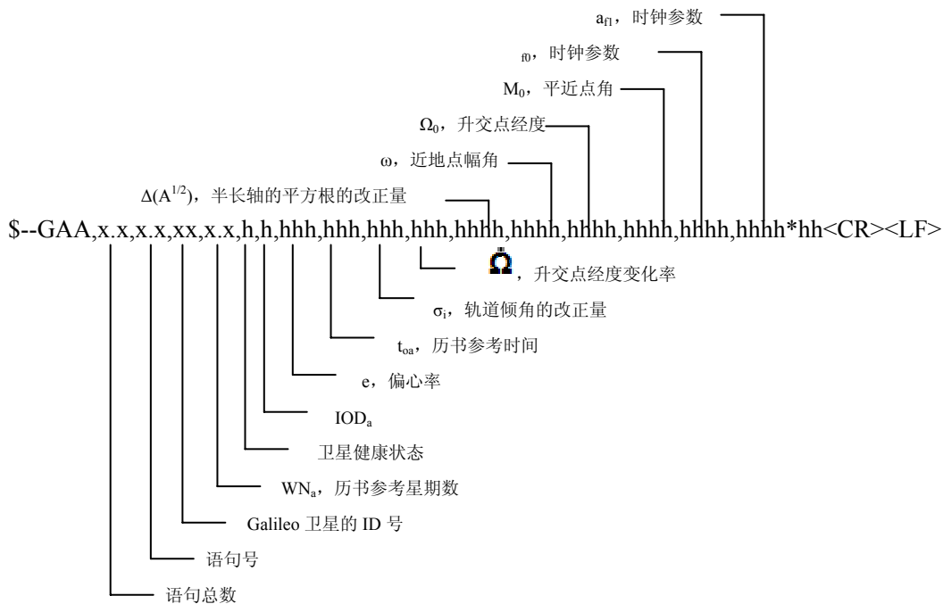
图 13 GAA—Galileo 历书数据语句说明
