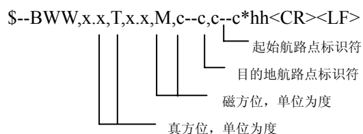
图 10 BWW 语句说明
