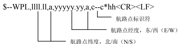
图 35 WPL 语句说明
