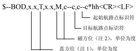
图 8 BOD 语句说明
