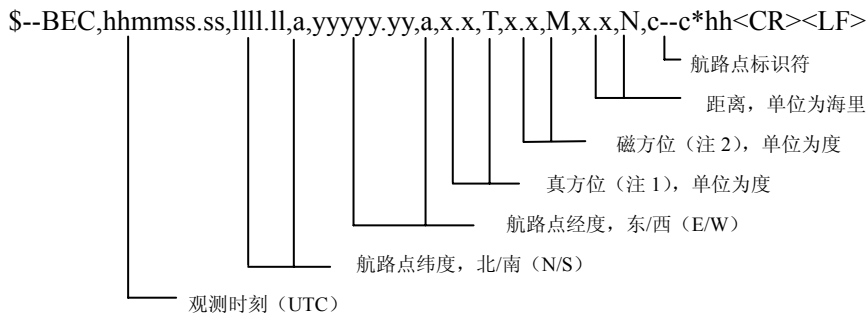
图 7 BEC 语句说明
