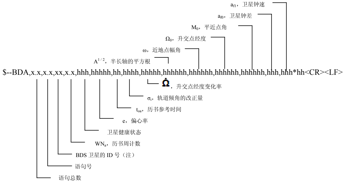
图 6 BDA—BDS 历书数据语句说明
