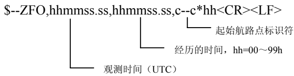
图 38 ZFO 语句说明
