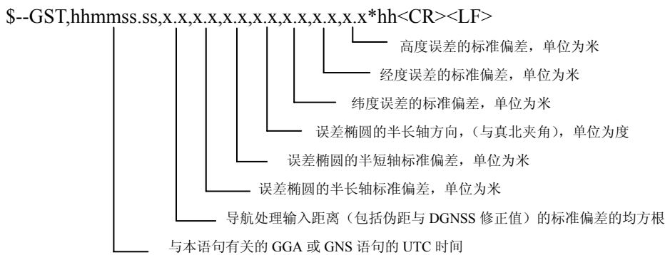
图 22 GST 语句说明
