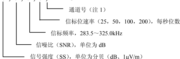
图 26 MSS 语句说明
