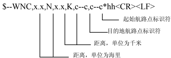
图 34 WNC 语句说明
