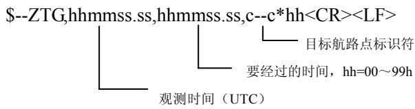
图 39 ZTG 语句说明
