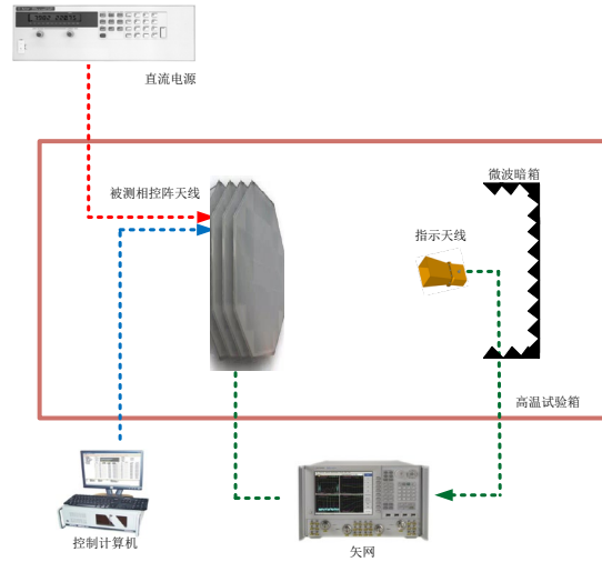
图 A.1 Ka 相控阵天线加速寿命试验设备连接框图示例
