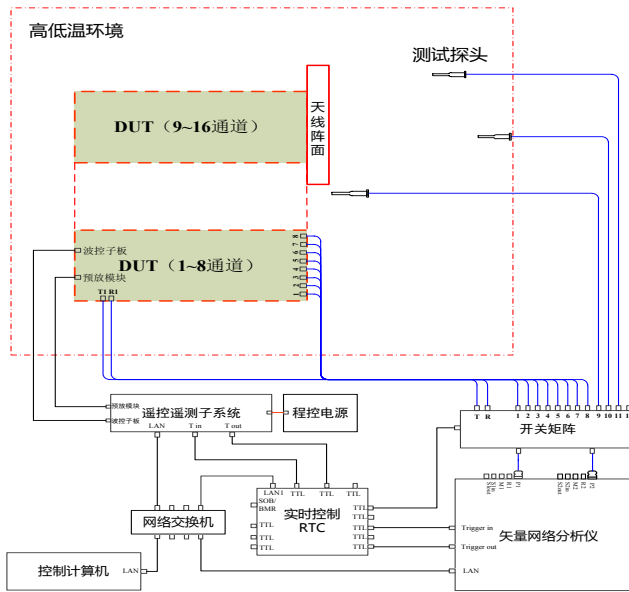
图 B.1 Ka 相控阵天线加速寿命试验设备连接框图示例
