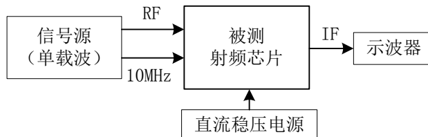
图 2 宽带射频芯片中频信号和采样时钟信号输出测试系统框图
