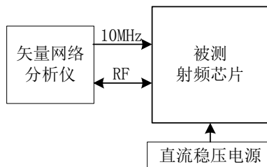
图 7 输入电压驻波比测试系统框图
