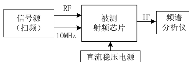
图 4 宽带射频芯片（扫频）测试系统框图
