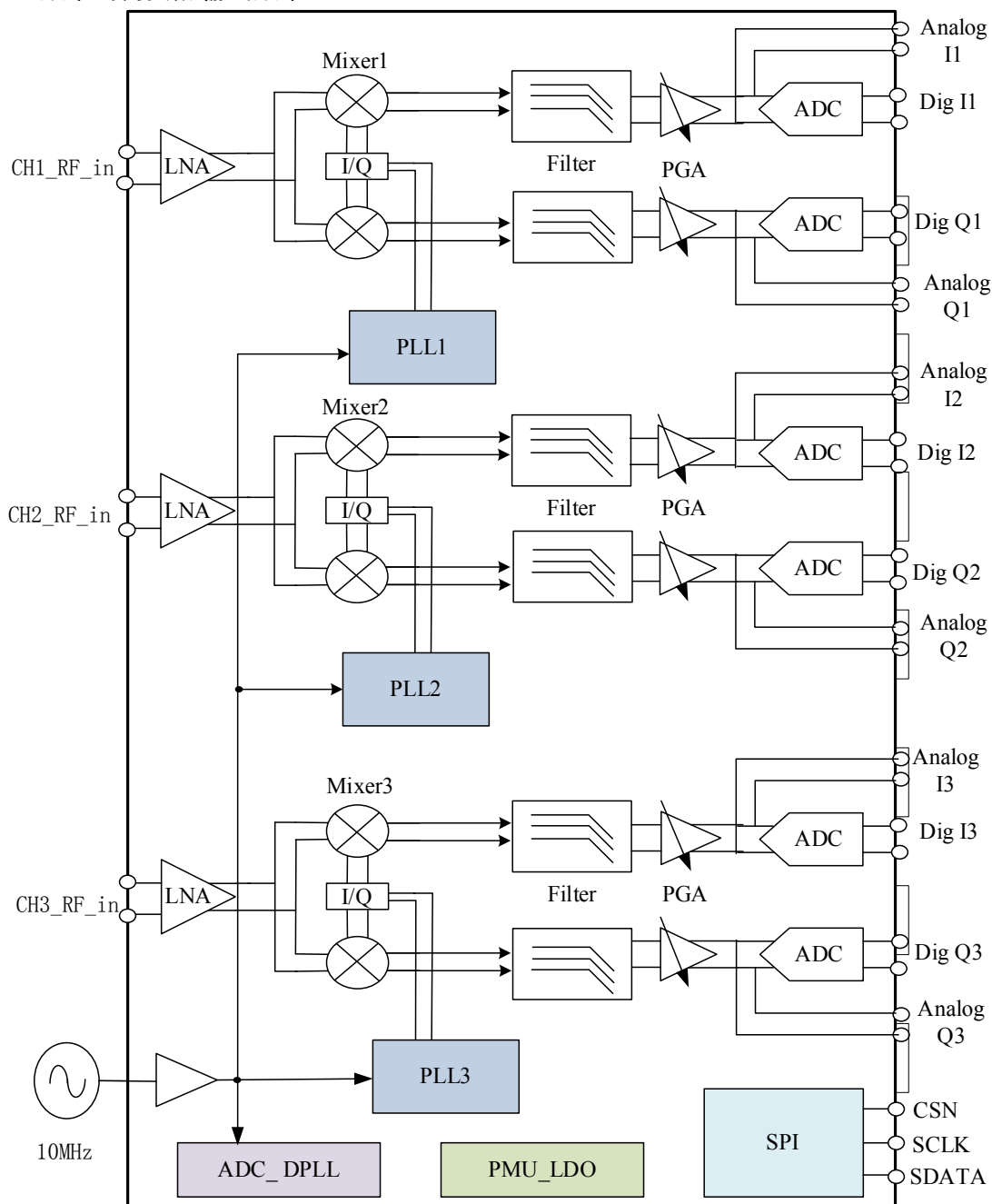
图1 宽带射频芯片系统组成示意图
