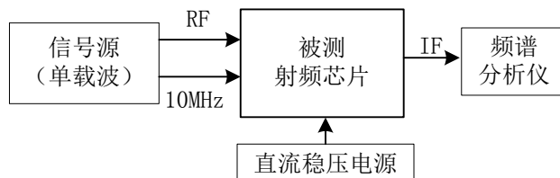
图 5 宽带射频芯片（单载波）测试系统框图
