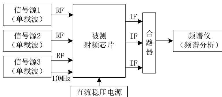
图 3 三通道并行工作测试系统框图
