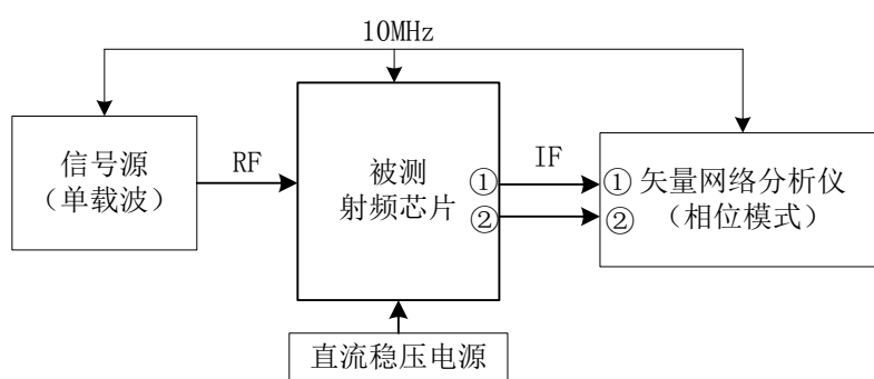
图 6 I/Q 适配相位误差测试系统框图
